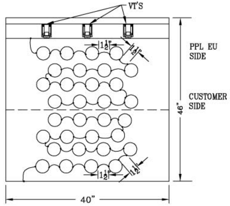
CONDUIT PLAN
